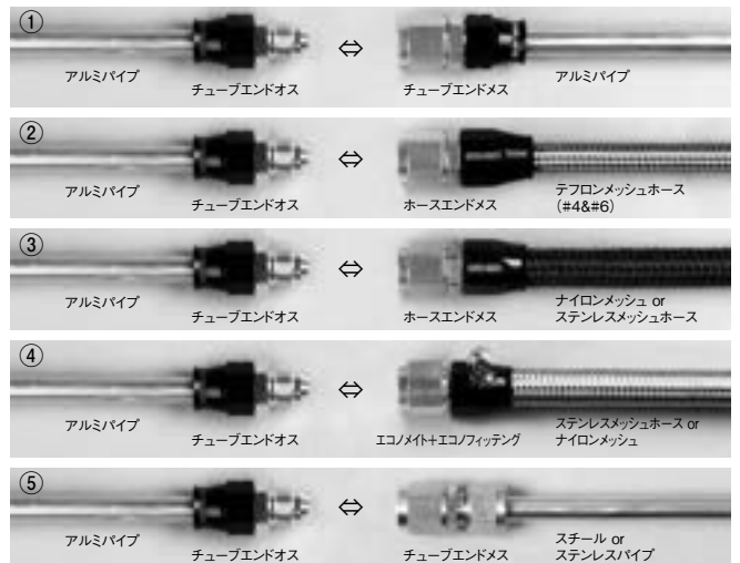
[チューブエンドオスタイプとその他の接続例]
