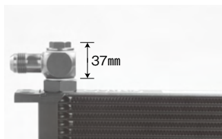
# 10 クーラーコアへの取り付け例 (横から)
