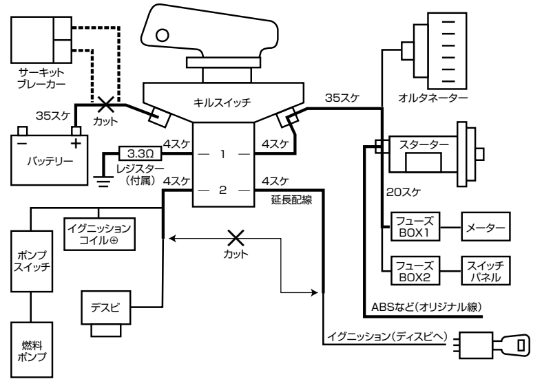
GE55 (配線図例)
