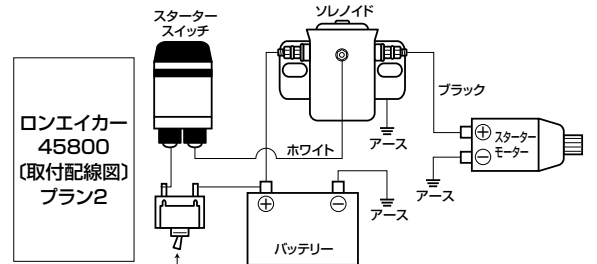
ON/OFFスイッチ類/イグニッションスイッチ (P350・P351 別売)
