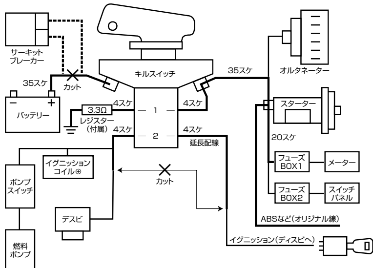
GE55 (配線図例)
