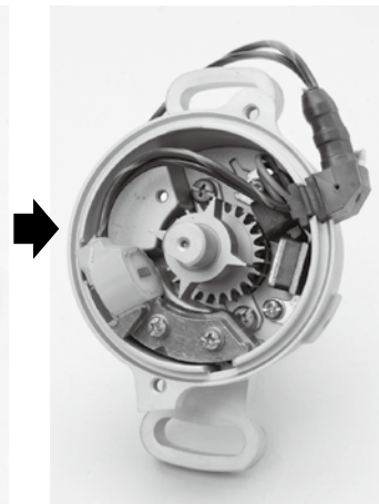
取り付け例
