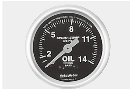
油圧計 ¥12,900 3322-K ●0~14Bar ●2"1/16(52φ)/56φ×D40mm ●ブラックパネル/ホワイトスケール
