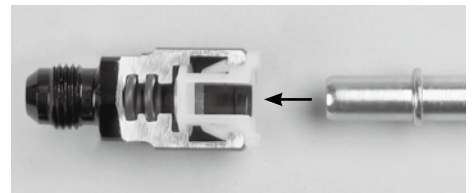
カット断面 ↓
